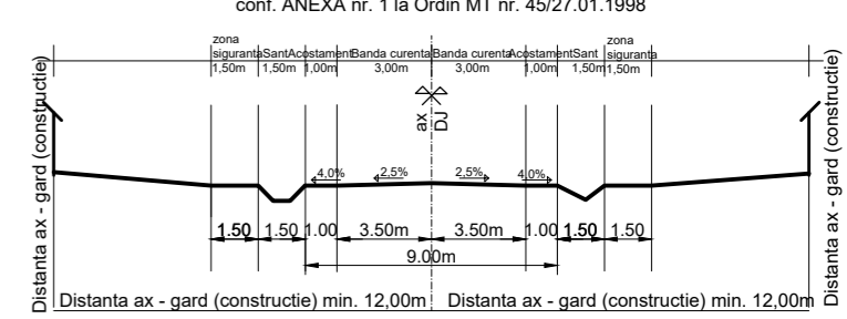
PROFIL 1 - 1 PROFIL TRANSVERSAL TIP DRUM JUDETEAN conf. ANEXA nr. 1 la Ordin MT nr. 4527/01.1998
