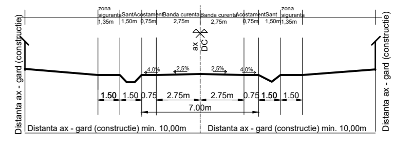
PROFIL 3 - 3 PROFIL TRANSVERSAL TIP DRUM SATESC conf. ANEXA nr. 1 la Ordin MT nr. 4527/01.1998
